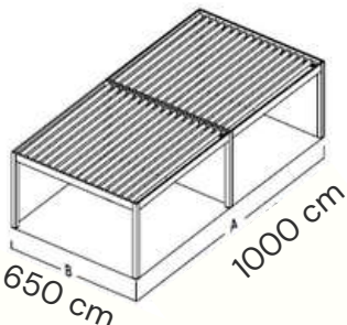
6 Piliers 650 x 1000 cm
