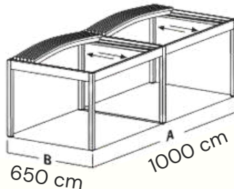
Taille maximum avec poutre AL2: A cm 1000 x B cm 650
