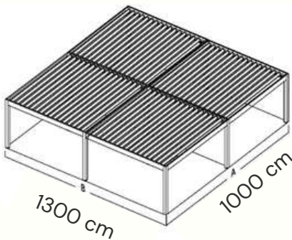
9 Piliers 1300 x 1000 cm
