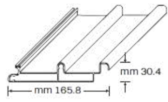
Lames réglables
