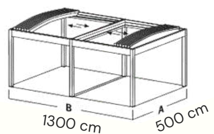
Taille maximum avec poutre AL2: A cm 500 x B cm 1300
