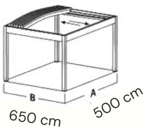
Taille maximum avec poutre AL2: A cm 500 x B cm 650
