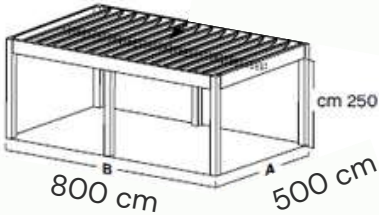
6 Piliers 500 x 800 cm
