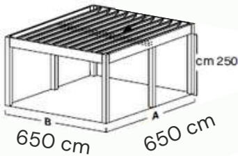
6 Piliers 650 x 650 cm
