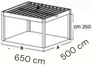
4 Piliers 500 x 650 cm
